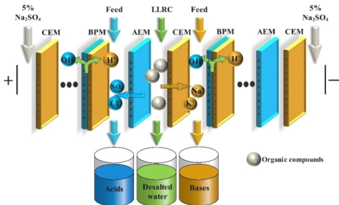
图2.双极膜电渗析的运行过程
