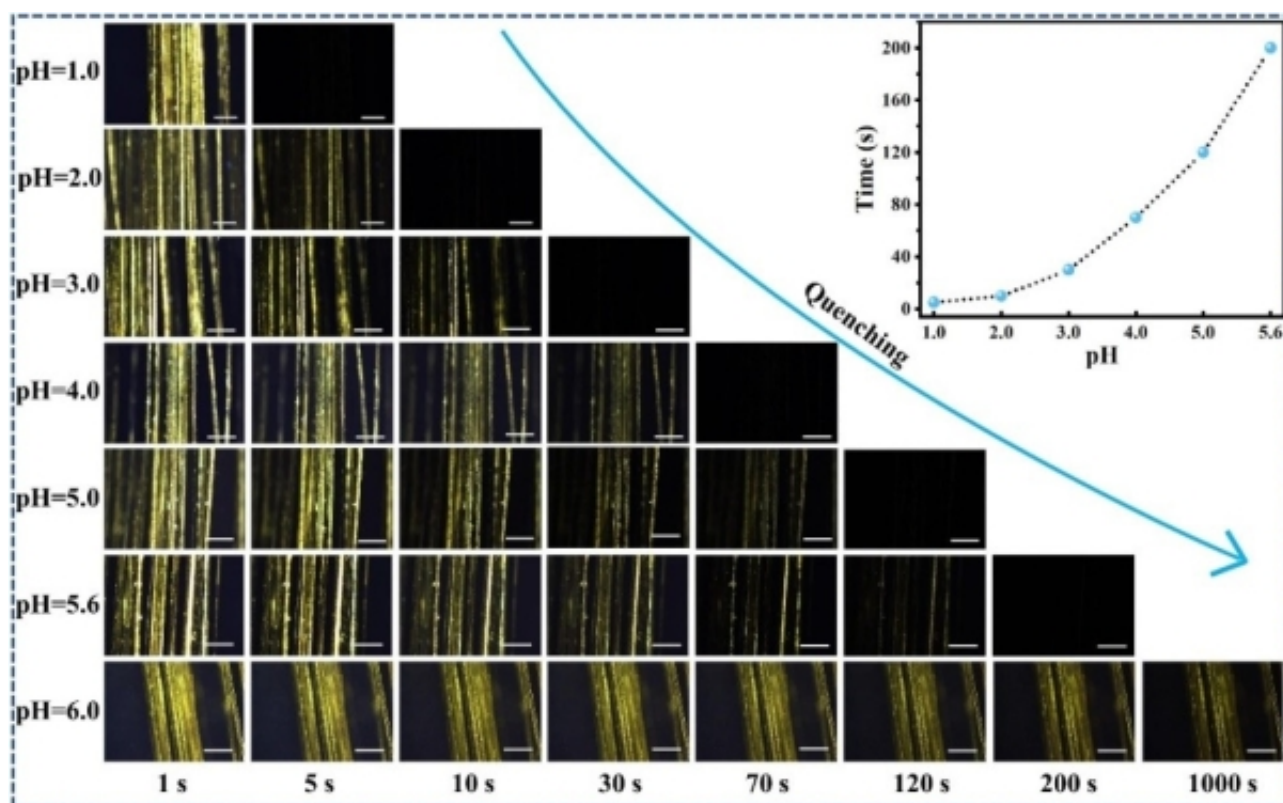
荧光玄武岩纤维及其应用(上图：具有不同荧光特性的玄武岩纤维;下图：不同pH溶液中黄色玄武岩纤维的荧光变化情况，插图为溶液pH值与荧光淬灭时间之间的关系)
