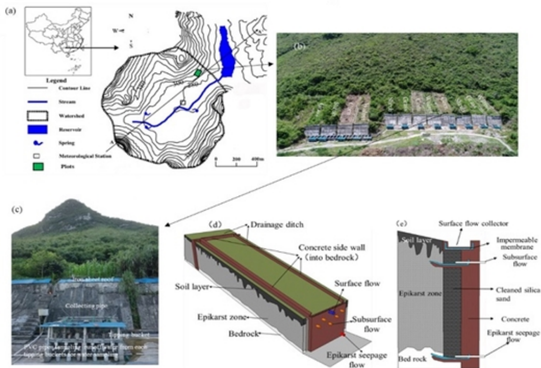
喀斯特坡地关键带多界面三维水土过程监测平台。受访者供图
