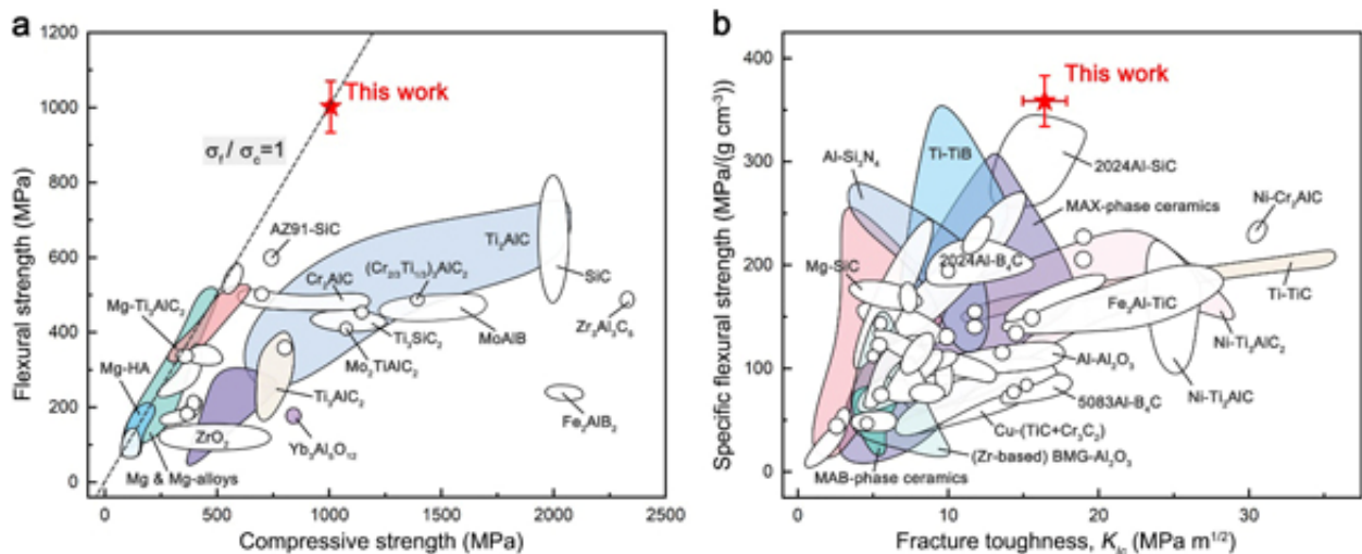
图2. 镁-MAX相仿生金属陶瓷的力学性能及其与其他材料的比较
