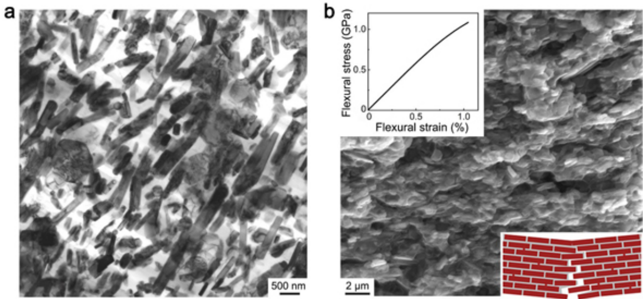
图1. 镁-MAX相仿生金属陶瓷的微观结构、弯曲力学性能与断裂机制
