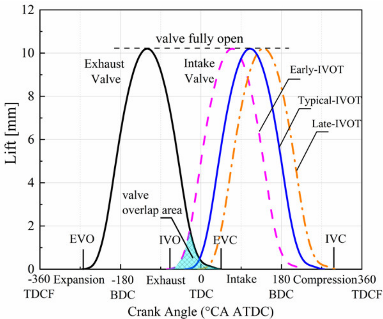
图2.变配气正时调控原理图
