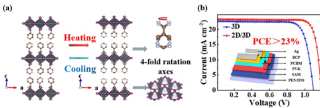
(a)新型二维钙钛矿的结构；(b)柔性器件的J-V曲
