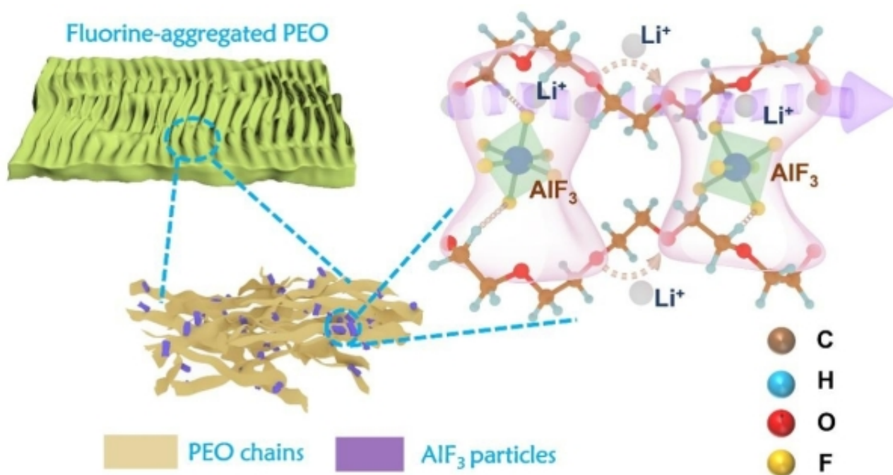
氟化PEO聚合物固态电解质的结构示意图
