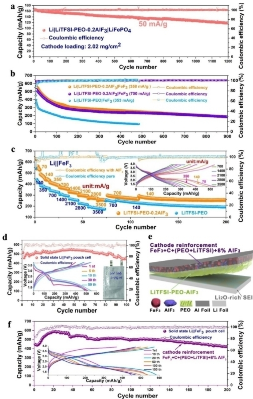
氟化增强的LiFeF 3 和LiLiFePO 4 固态电池的电化学性能
