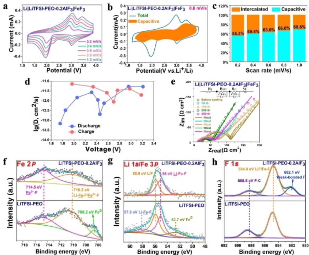
LiFeF 3 固态电池的动力学性能和循环后正极侧的表面组分
