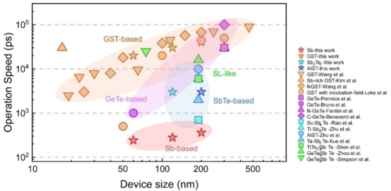
图2 单质锑相变存储器操作速度与已报道相变存储器件的对比
