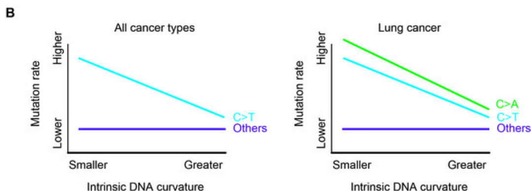
图：DNA固有曲率调控局部突变率。(A) DNA固有曲率能够降低突变率机制的示意图。(B) DNA固有曲率抑制了所有癌症及肿瘤类型共有的(C>T)和肺癌特异的(C>A)由诱变剂诱导的突变。
