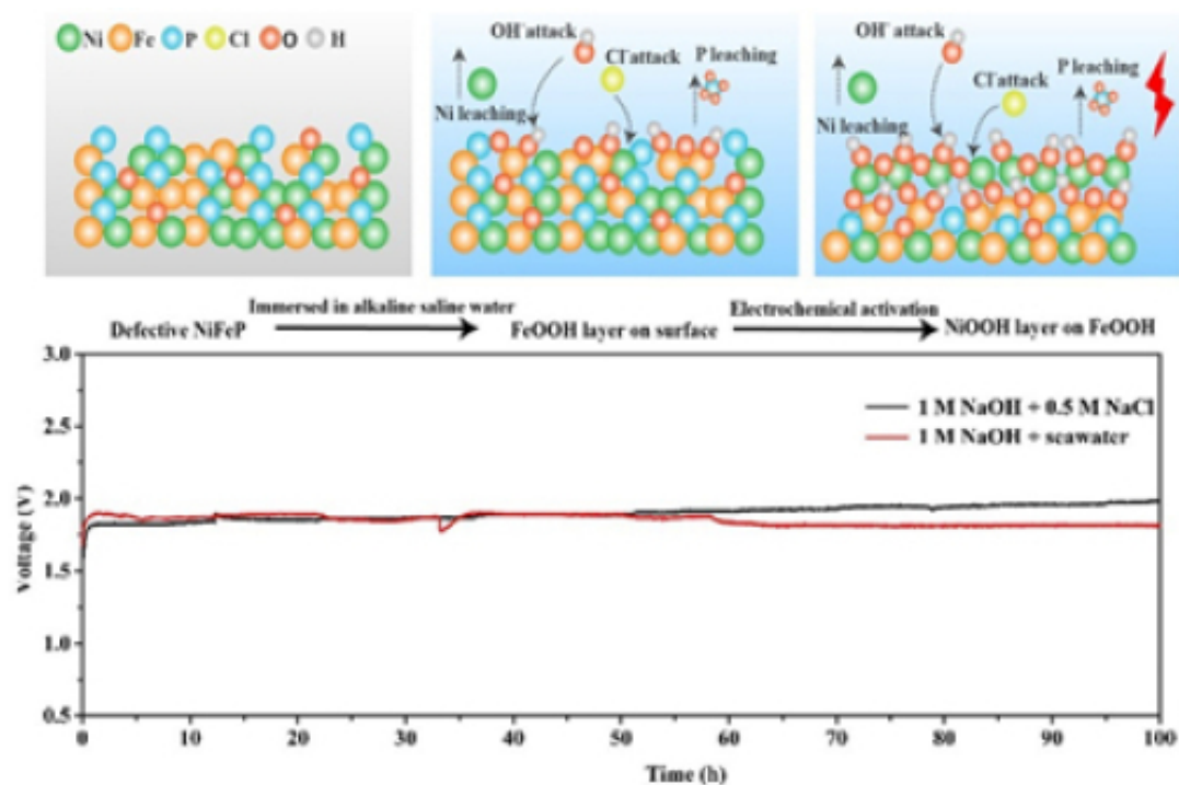
图1. NiOOH@FeOOH 异质结构和海水电解 OER 性能
