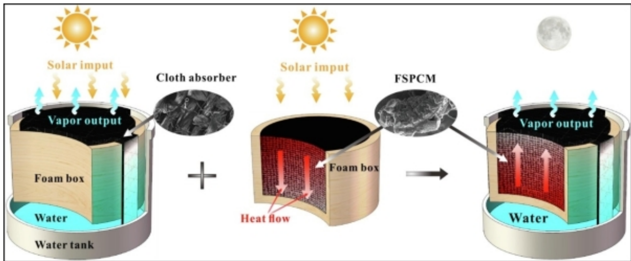
相变蓄热材料强化太阳能界面水蒸发系统工作模式图
