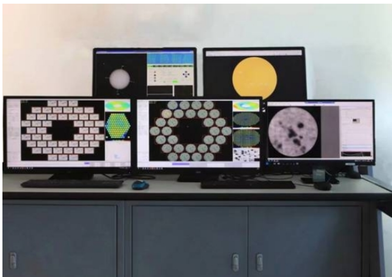
图1.太阳多层共轭自适应光学系统实物照片
