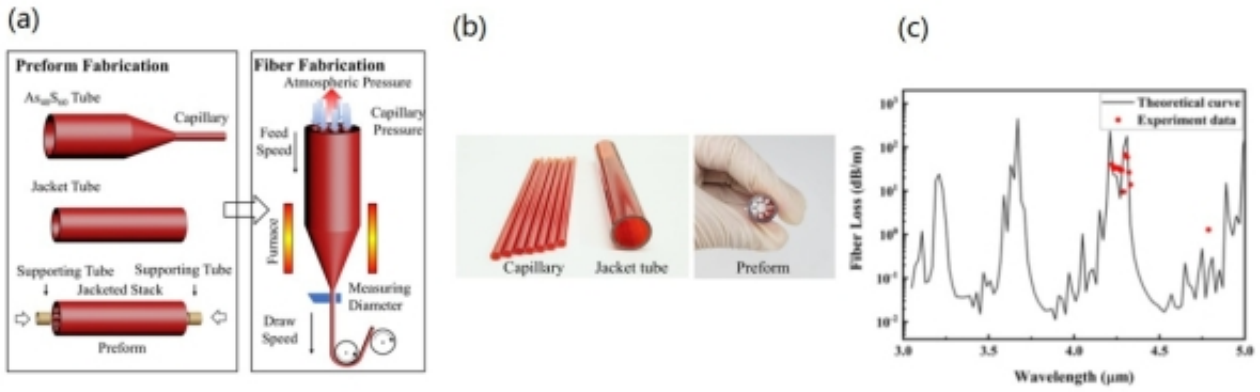
(a) 堆积拉制法和双路气压控制技术 (b) 光纤预制棒 (c) 光纤的理论损耗与实测损耗
