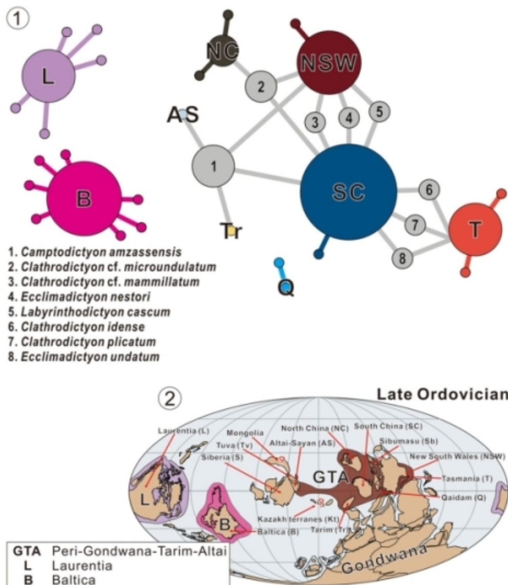
图1.华南晚奥陶世层孔海绵的网络分析及生物古地理区系
