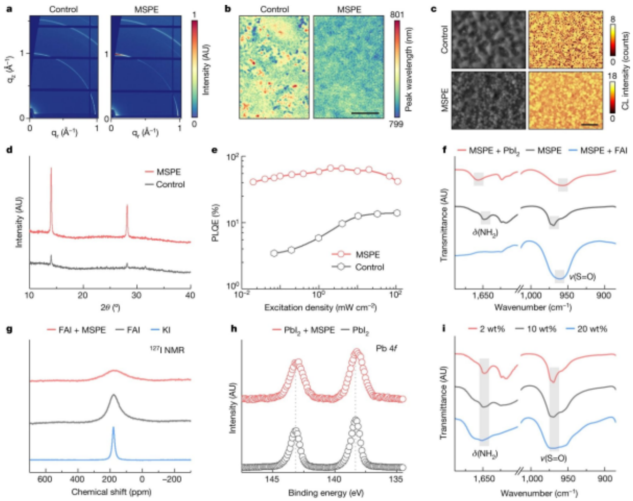
图2. 钙钛矿薄膜以及分子间作用的表征
