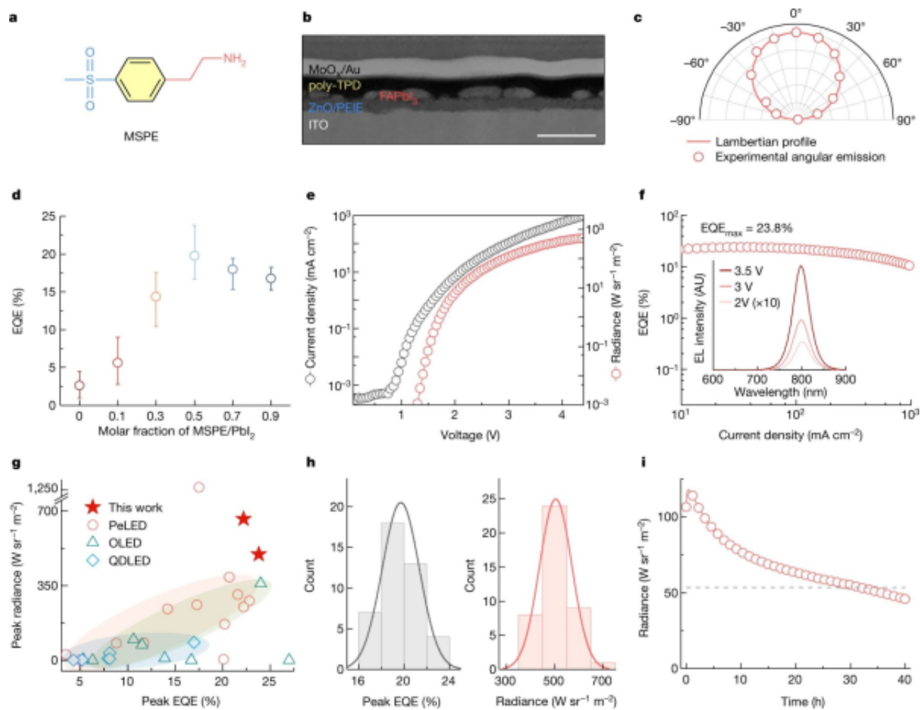
图1.钙钛矿LED结构和性能
