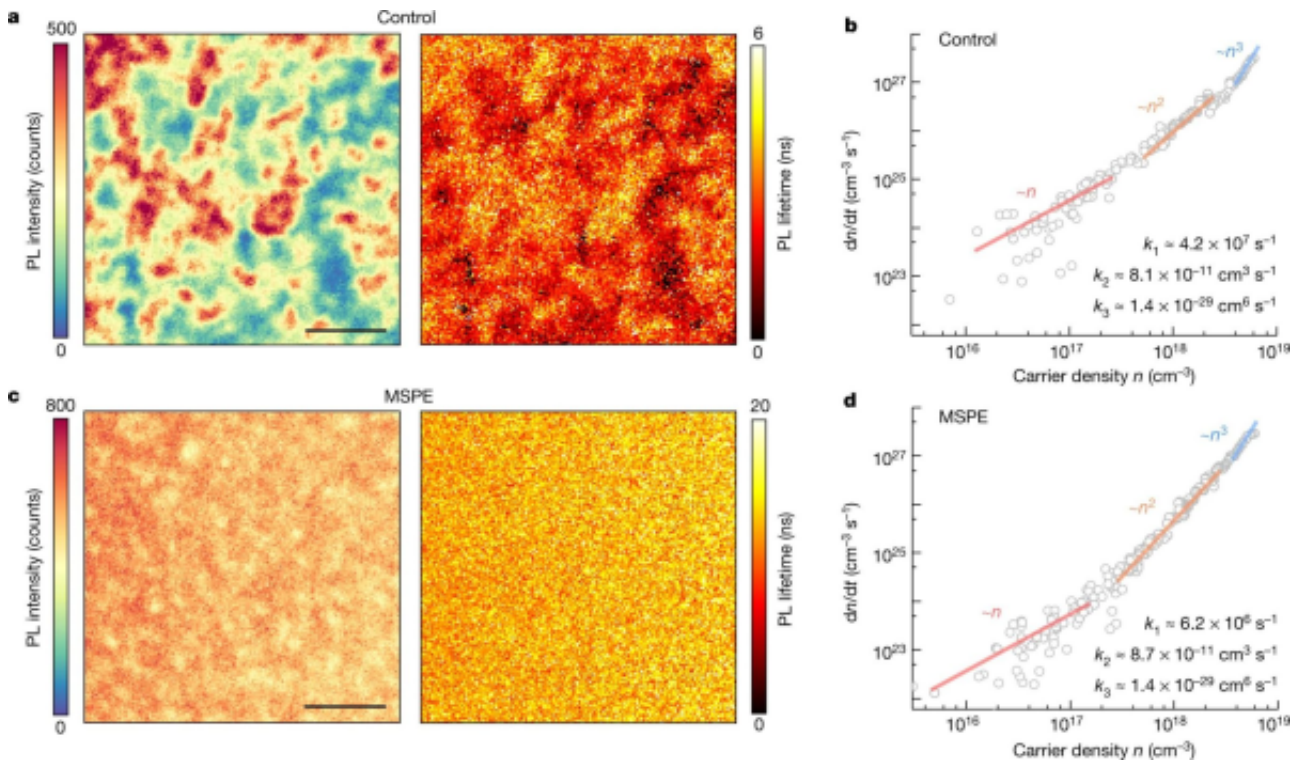
图3.钙钛矿薄膜的载流子动力学
