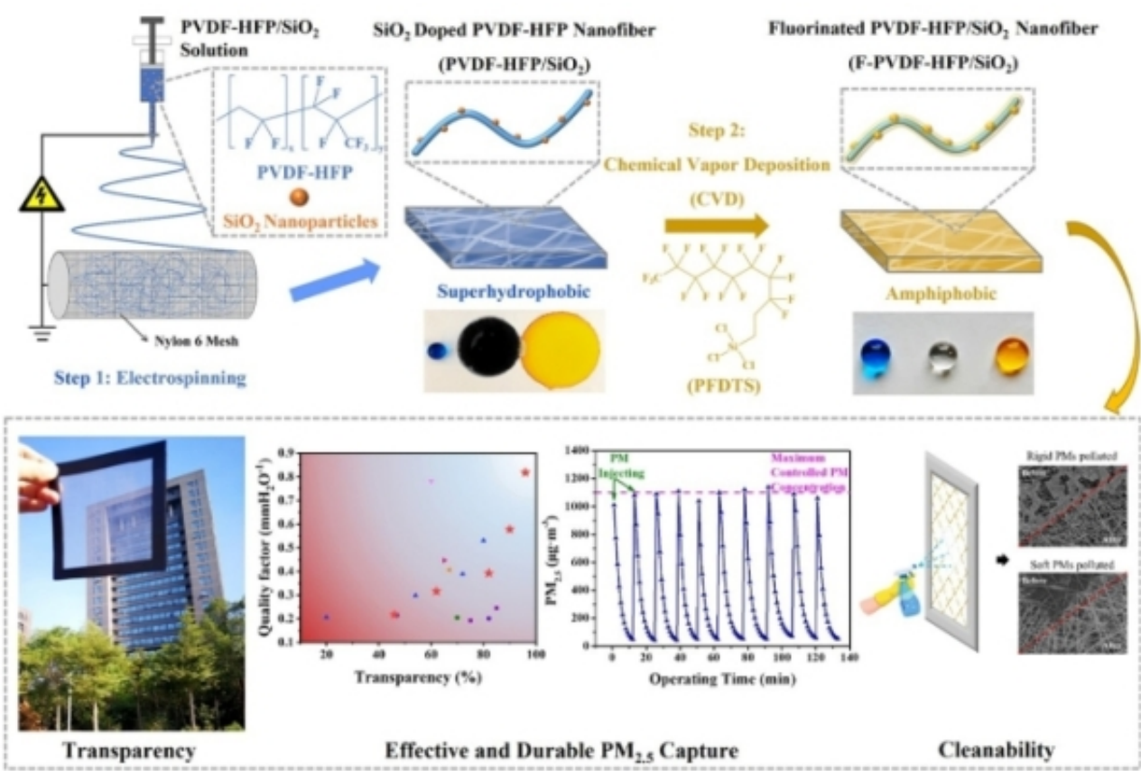
可清洗的透光防霾纱窗的制备及其性能表征
