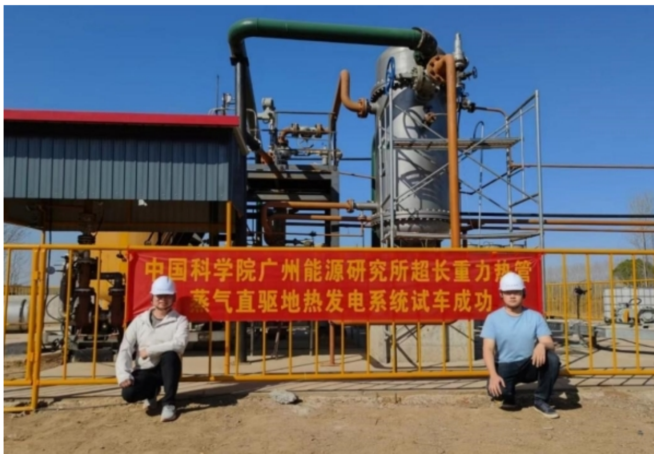
SLGHP蒸气直驱地热发电系统试验现场
