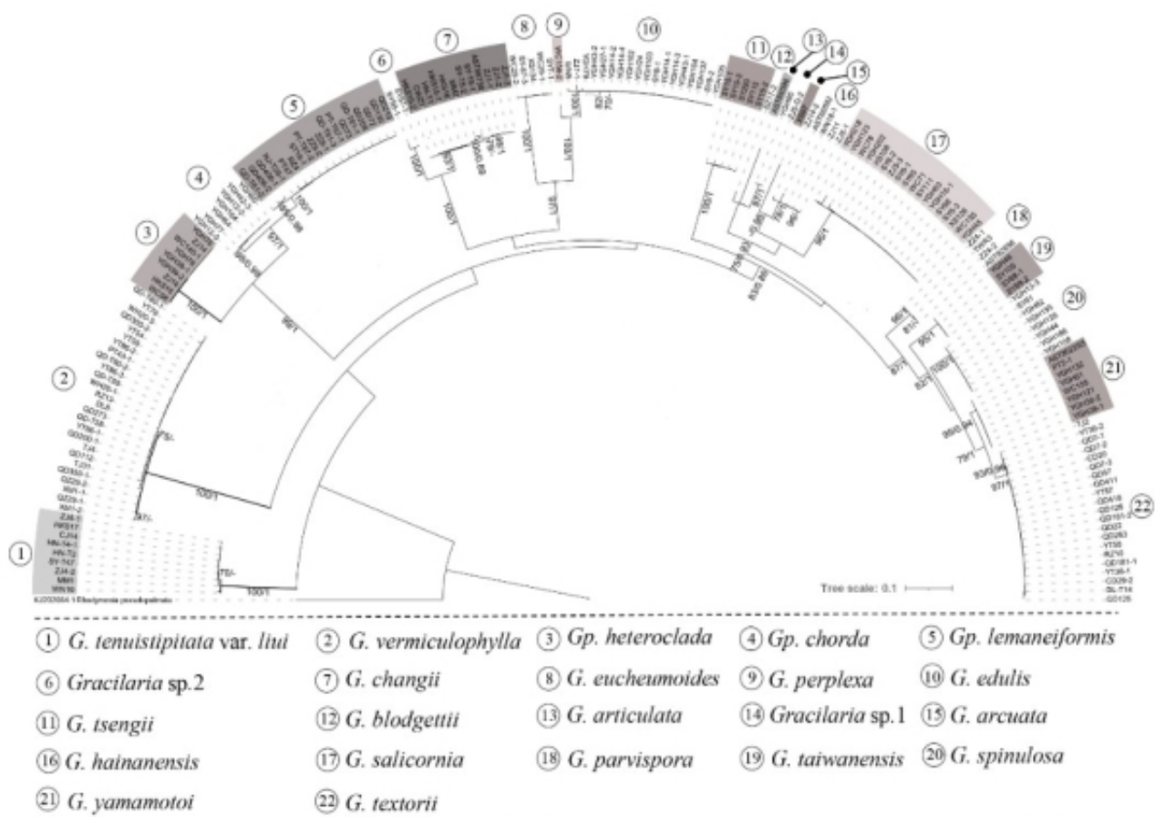
基于rbcL数据集构建的我国江蓠科物种系统发育树
