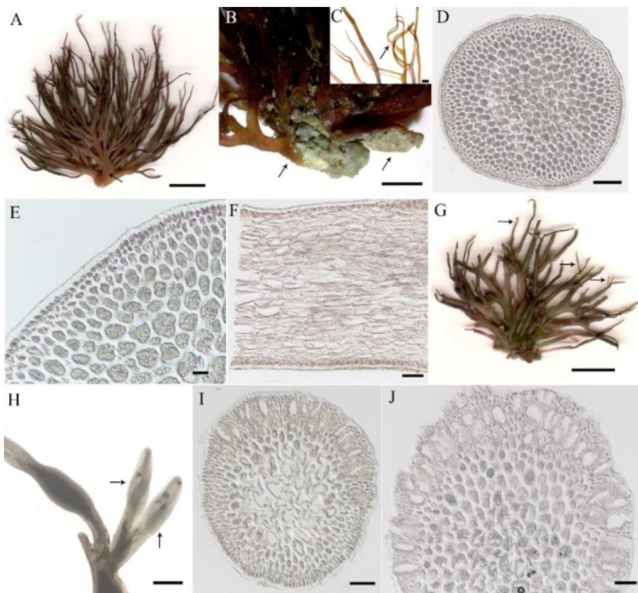
曾氏江蓠外部形态、内部构造及其精子囊枝（标尺：A/G、0.5 cm；B、1 mm；C、500 \mu\text{m} ；D、100 \mu\text{m} ；E、20 \mu\text{m} ；F/I/J、50 \mu\text{m} ；H、400 \mu\text{m} ）
