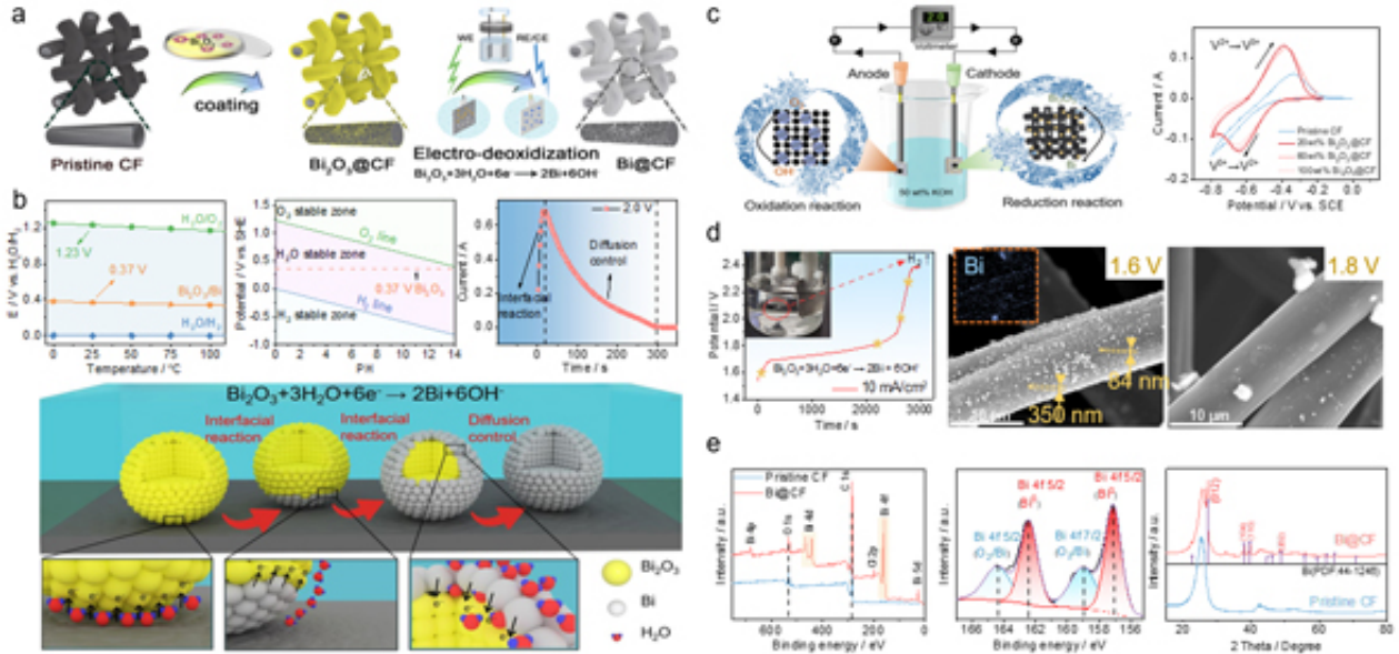
图3.(a)电脱氧制备工艺;(b)热力学计算和脱氧反应机理;(c)电解池示意图及循环伏安曲线图;(d)还原电位及表面形貌图;(e)电极成分表征。
