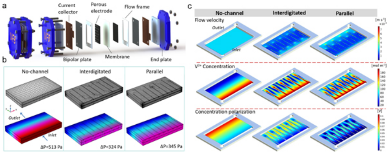
图1.(a)电池结构示意图;(b)电池压降仿真;(c)流速、反应物浓度及浓差极化分布仿真。
