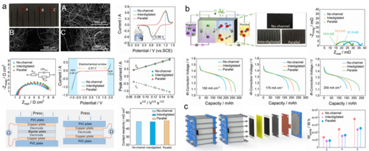
图2.(a)电极物理及电化学测试;(b)全钒液流电池实验;(c)电堆动态模拟。
