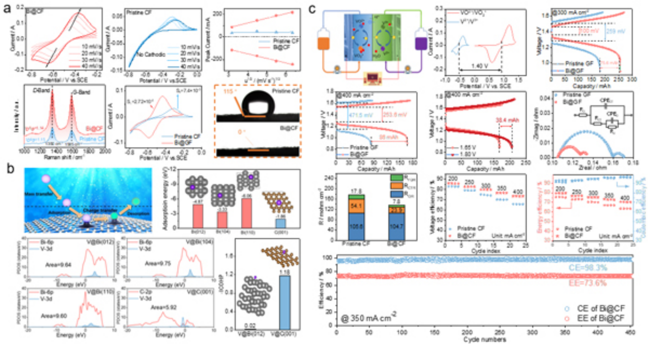
图4.(a)电极物理及电化学表征;(b)界面电化学理论计算;(c)全钒液流电池实验。
