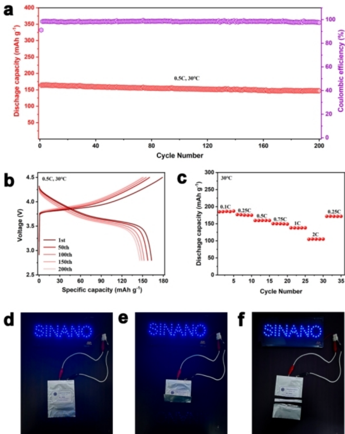
图3. LiP(IL-OFHDODA-VEC)NCM523全电池的电化学性能。a. LiP(IL-OFHDODA-VEC)NCM523全电池在0.5 C下的循环性能；b. LiP(IL-OFHDODA-VEC)NCM523全电池的第1-200次充放电曲线；c. LiP(IL-OFHDODA-VEC)NCM523全电池的倍率性能；d-f. 充满电的LiP(IL-OFHDODA-VEC)NCM523软包电池在折叠前 (d) 和折叠后 (e) 或切割后 (f) 点亮LED灯的照片。
