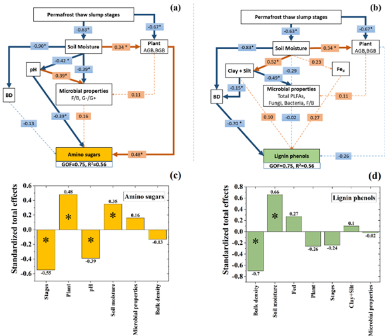
图3.最小二乘路径模型模拟结果
