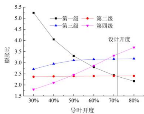
(d) 膨胀比与导叶开度之间的关系
