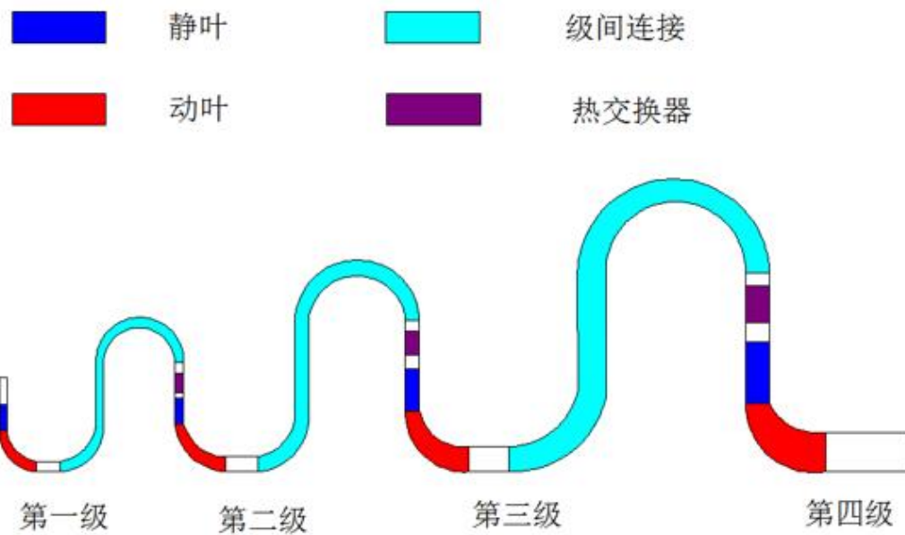
图1多级再热向心透平模拟示意图
