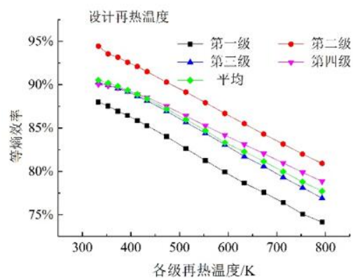
(c) 等熵效率与再热温度之间的关系
