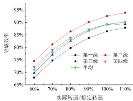
(b) 等熵效率与转速之间的关系
