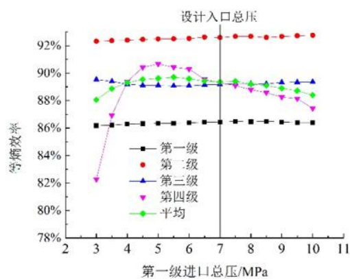
(a) 等熵效率与进口总压之间的关系
