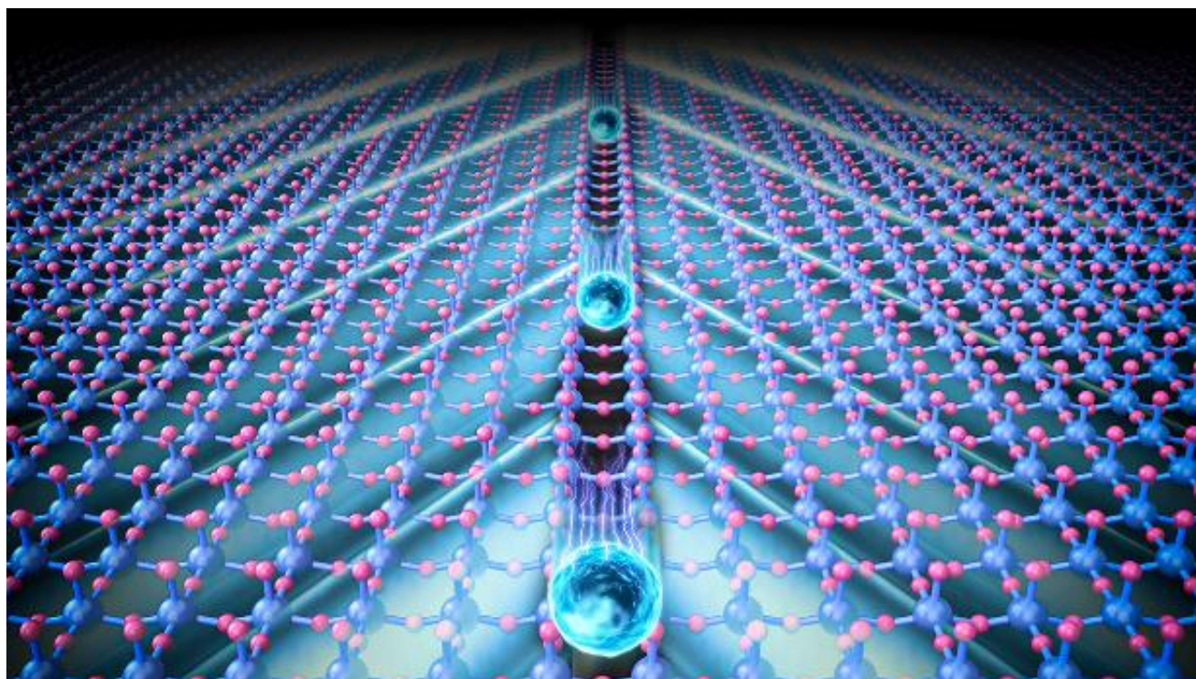
极化激元反向切伦科夫辐射的示意图(研究团队供图)
