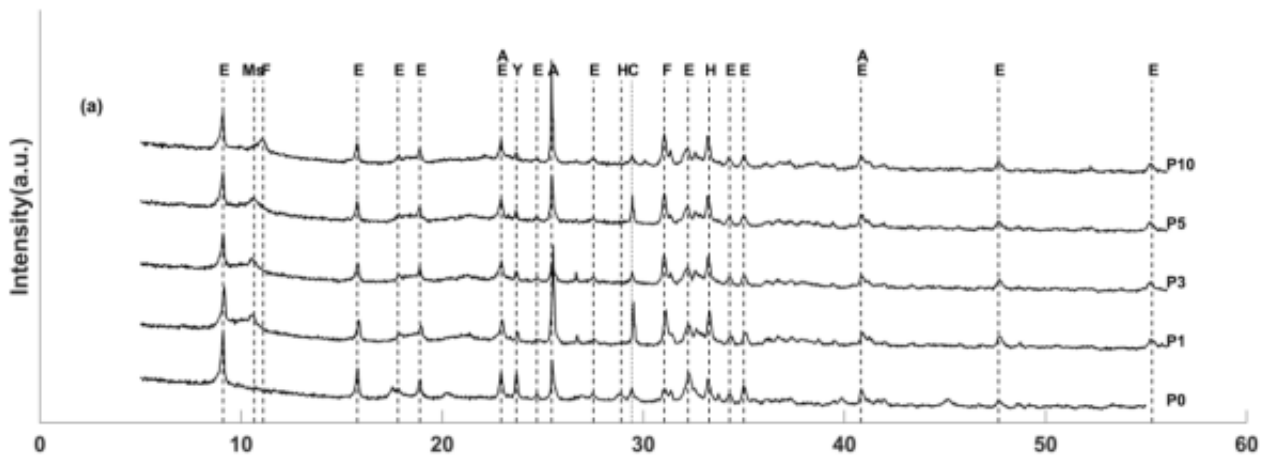
图2不同海水盐浓度下水化产物的演化
