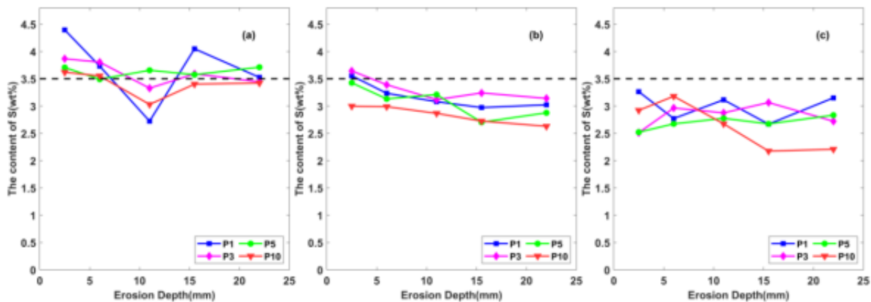
图3 不同盐浓度与腐蚀龄期下材料体系中硫元素含量的变化过程(a) 0.5a, (b) 1.0a, (c) 1.5a
