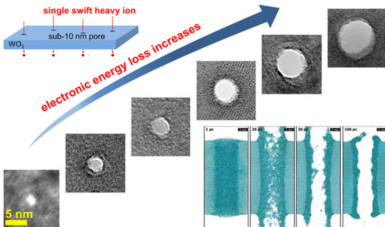
快重离子在WO 3 纳米片中直接形成纳米孔示例。近物所供图
