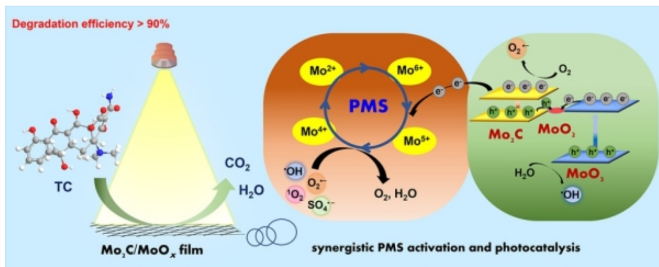
图2. 新型钼基纳米异质结光催化/PMS氧化偶联体系
