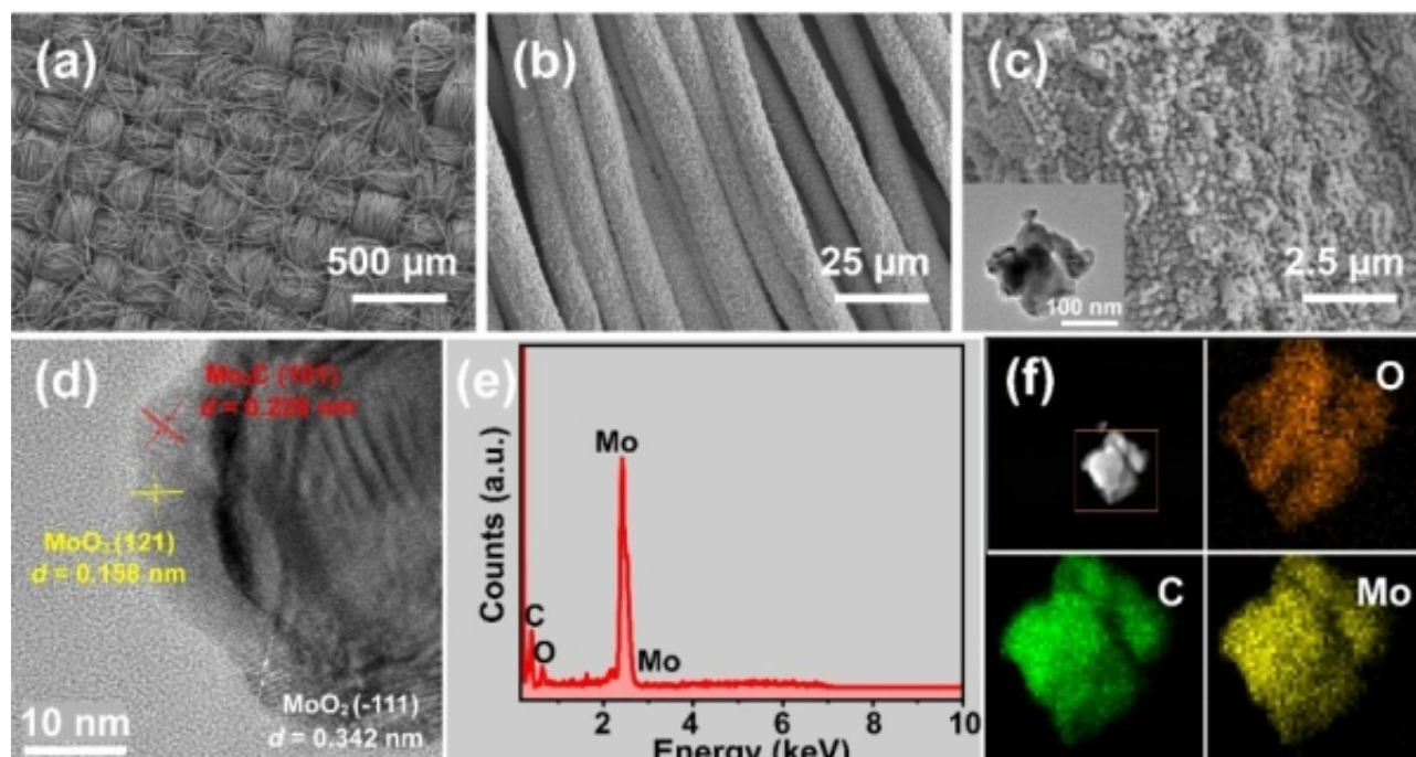
图1. 钼基纳米异质结构(Mo 2 C/MoO x )
