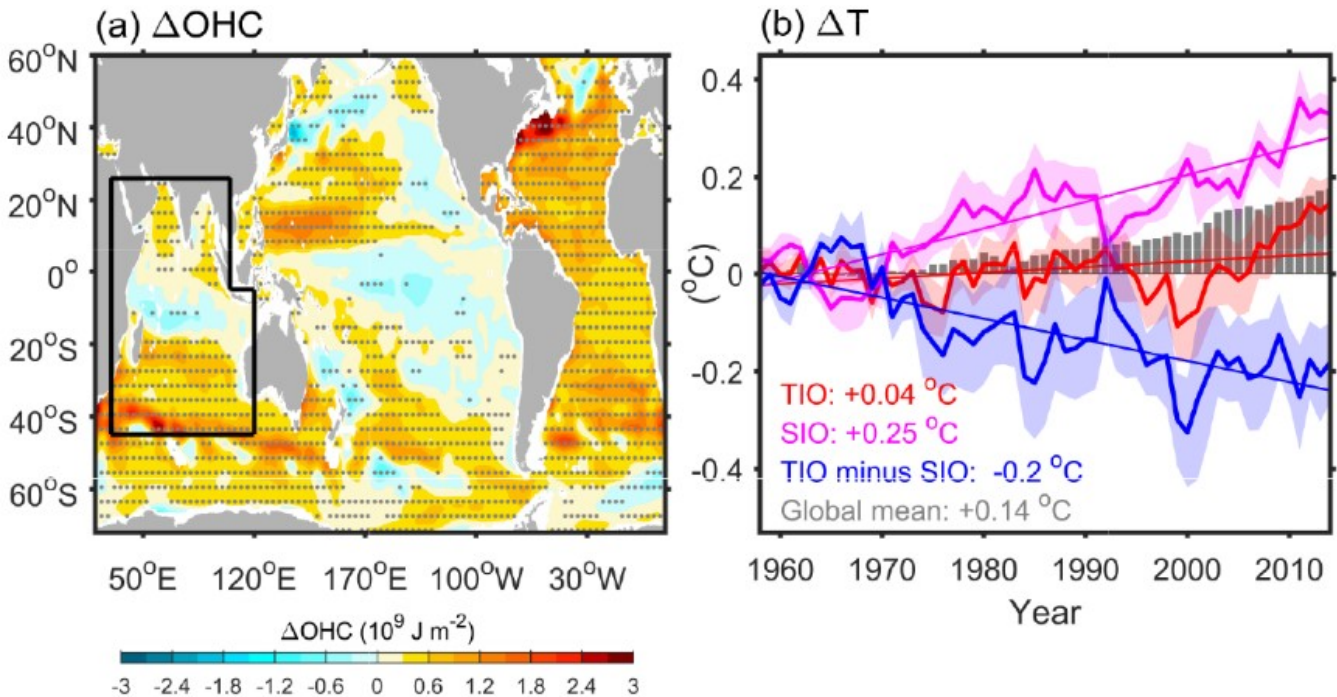
观测集合平均在1958-2014年期间0-700米的海洋热含量变化 海洋研究所供图
