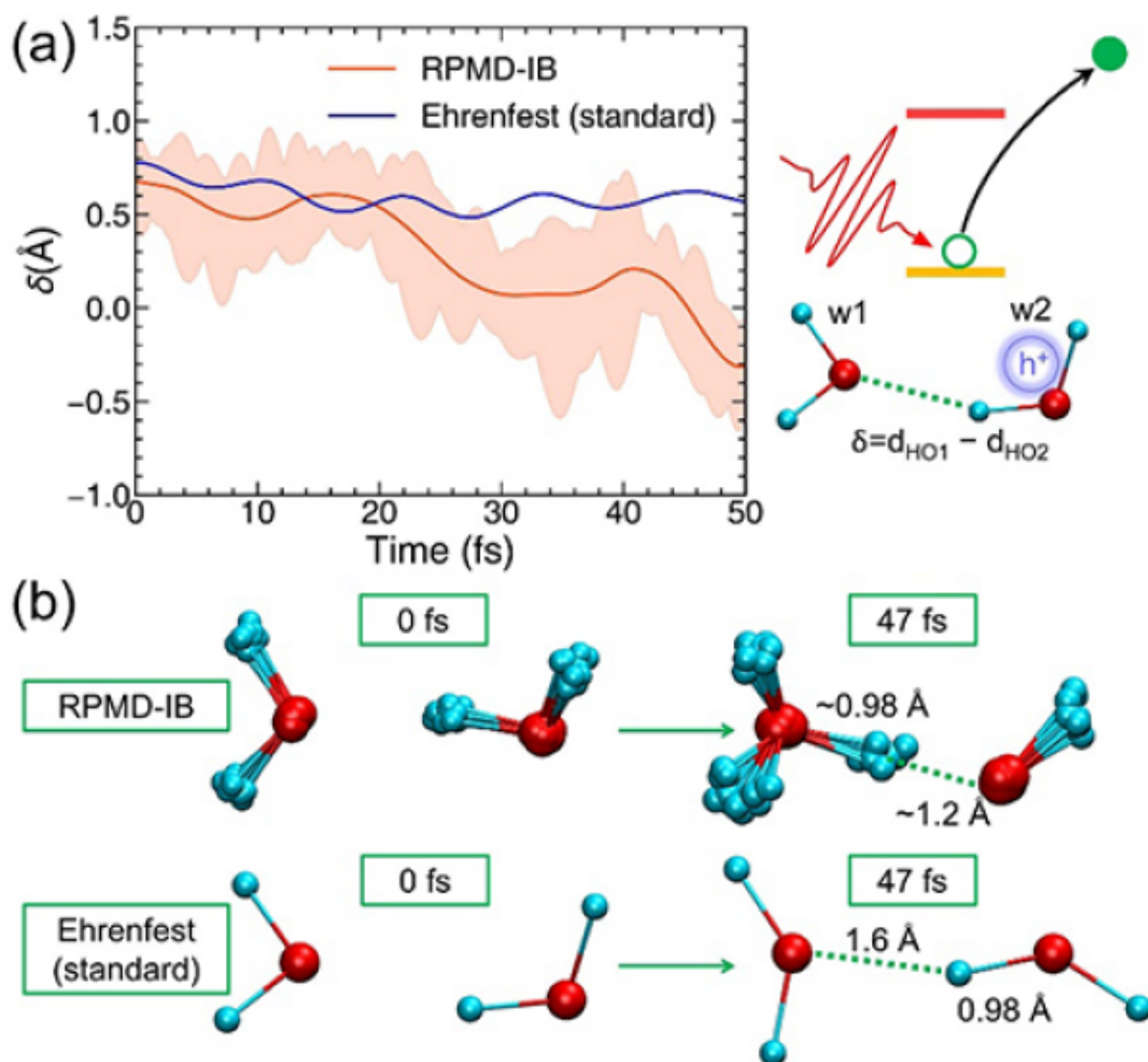
图4. RPMD-IB方法与传统Ehrenfest平均场方法模拟H 2 O-H 2 O + 中质子转移过程的对比。(a)质子在水分子二聚体中位置随时间的变化，(b)不同时刻水分子二聚体空间结构对比。
