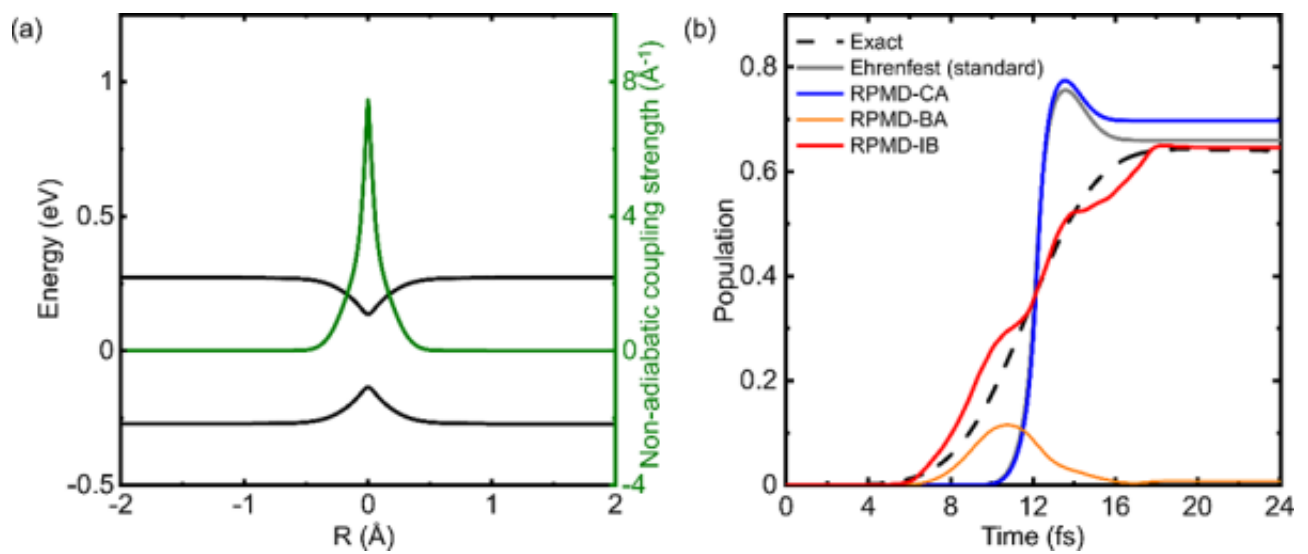
图2. 新发展的RPMD-IB方法在二能级模型中的结果。(a)二能级模型中的势能面(黑线)与非绝热耦合量(绿线)。(b)在不同方法中，电子在高能级的占据数随时间的变化。虚线为量子力学严格解。
