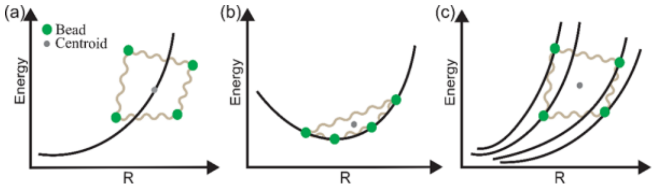
图1. 几种非绝热路径积分分子动力学方法图示。(a)RPMD-CA , (b) RPMD-BA , (c) RPMD-IB。
