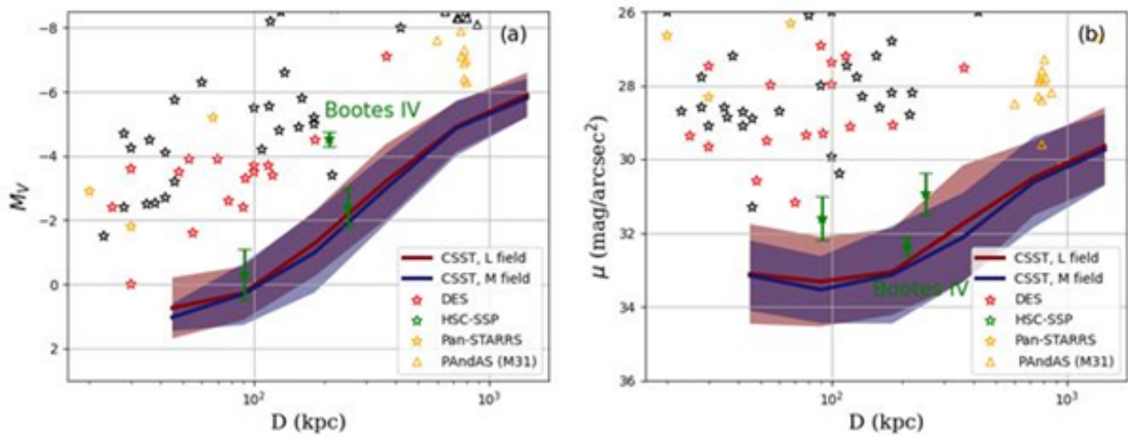
图3. CSST矮星系探测极限与已有的MW、M31卫星星系分布对比，星号与三角形分别标记了在各个巡天项目中首次被探测到的MW与M31的卫星星系。
