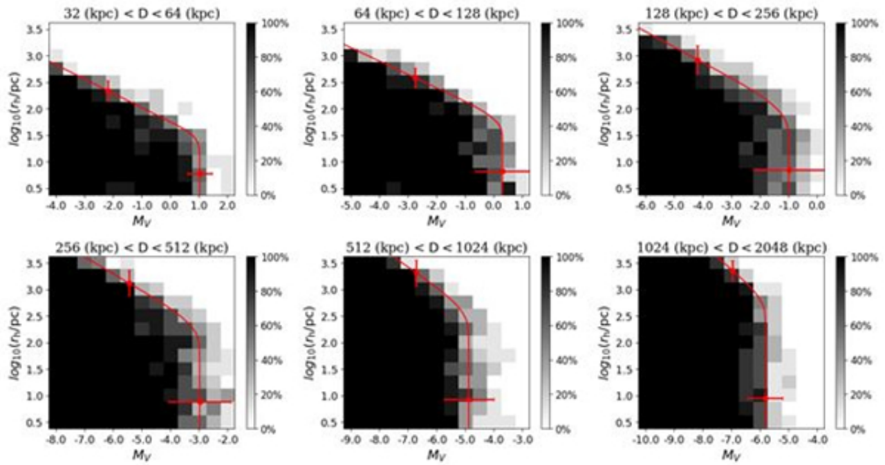
图2. CSST主巡天中银纬 ( b : 30\sim60 ) 区域不同距离、亮度与半光半径的矮星系探测成功率分布。
