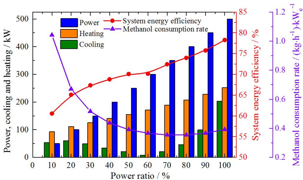
图2.化学回热过程T-Q分析及分布式供能系统变工况性能(白章, 刘启斌等, Applied Energy, 2018)
