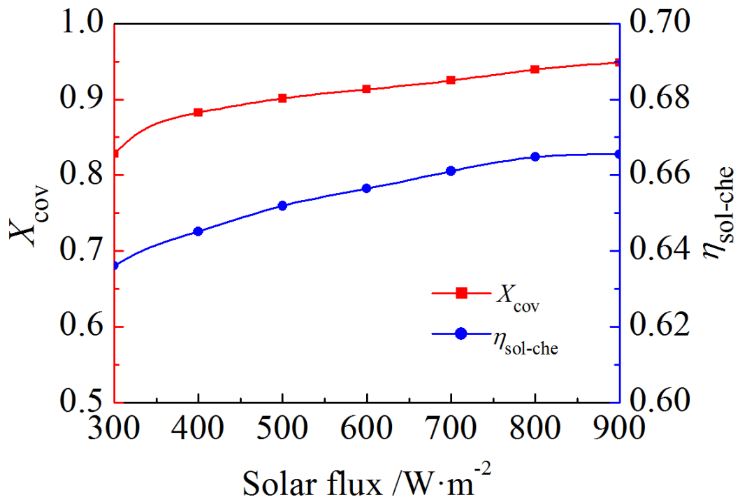
图1.太阳能热化学燃料转化结构形式与其热力学性能(刘泰秀, 刘启斌等, AppliedEnergy, 2018)
