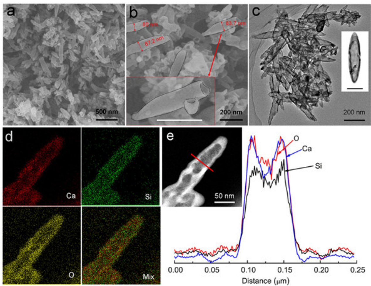
图3. (a) 样品的制备过程, (b) 合成样品的SEM和 (c) TEM图像, (d) Ca 80 Mg 20 复合吸附剂的FESEM和各元素分布的Mapping图像
