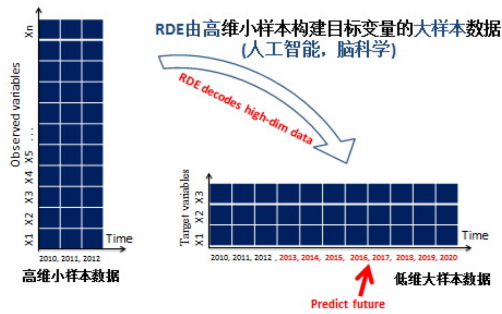
图1 随机嵌入分布方法转换高维数据为目标变量(低维)的动态信息，实现短序列数据的预测，同时RDE可看作是由高维小样本构建目标变量的大样本数据方法
