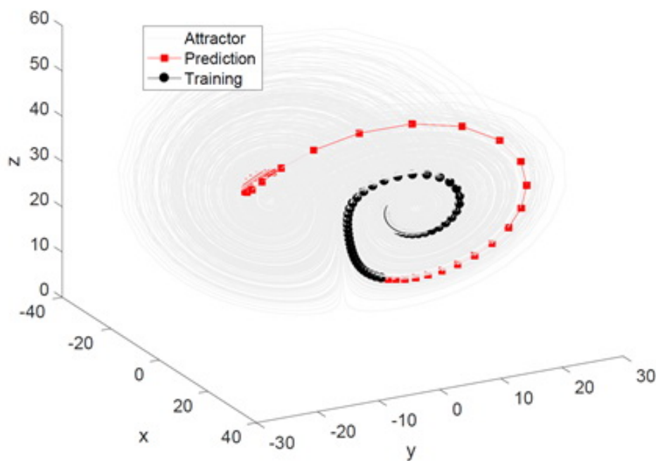
即使学习数据只是吸引子的一部分样本(黑色)，但RDE可预测那些没有学习过的动态行为(红色)
