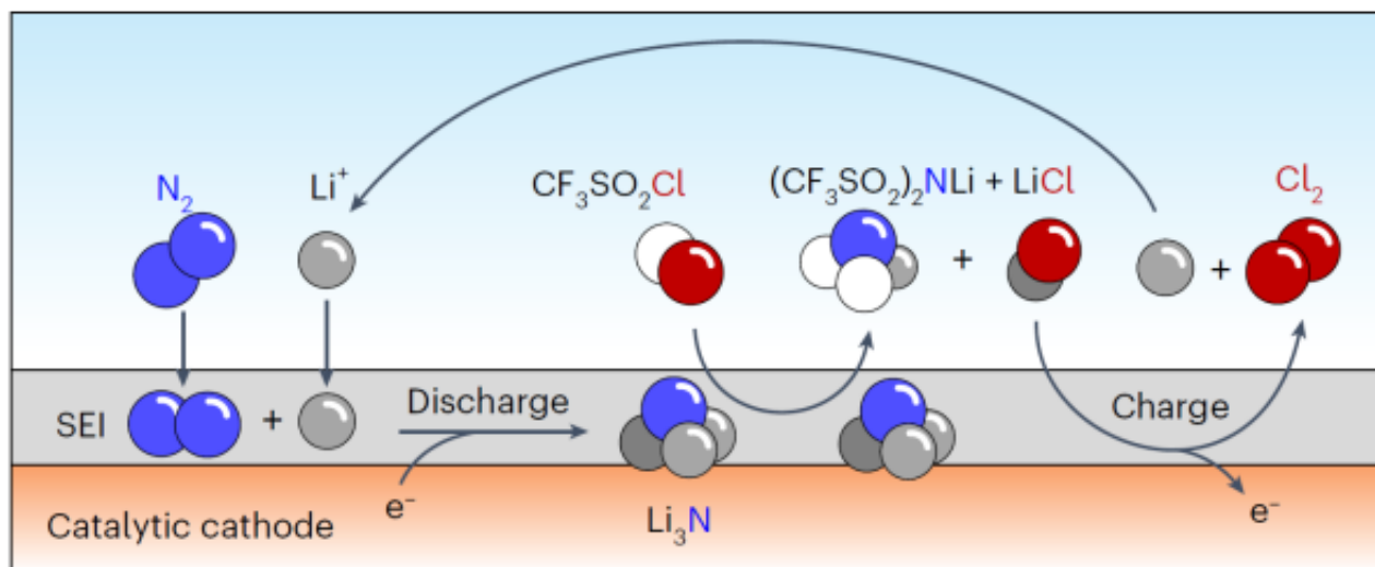
Li-N 2 电池电化学合成LiTFSI的级联反应示意图
