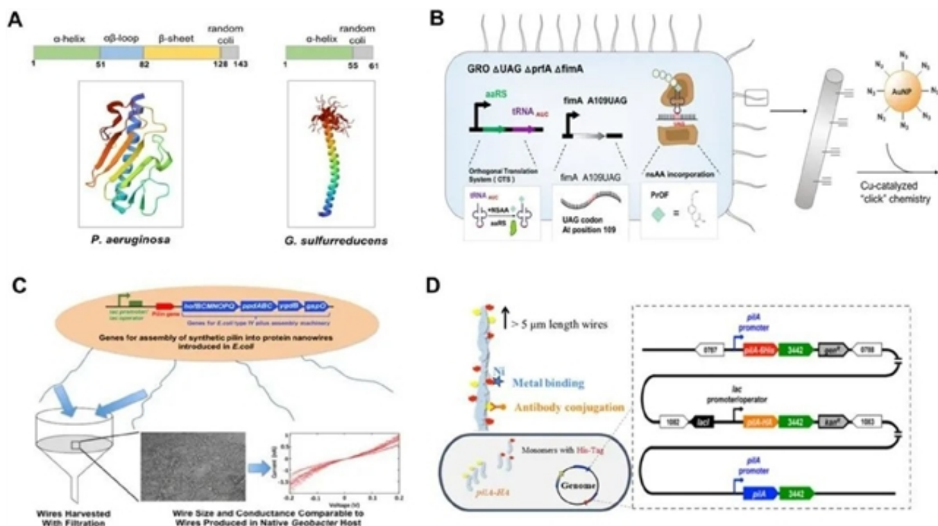
图3. 工程改造导电纳米线 A. PaPilA和GsPilA的三级结构和序列图；B. 高电导率pilin纳米线的工程设计；C. 大肠杆菌中异源合成e-pili；D. 利用短肽修饰e-pili表面。
