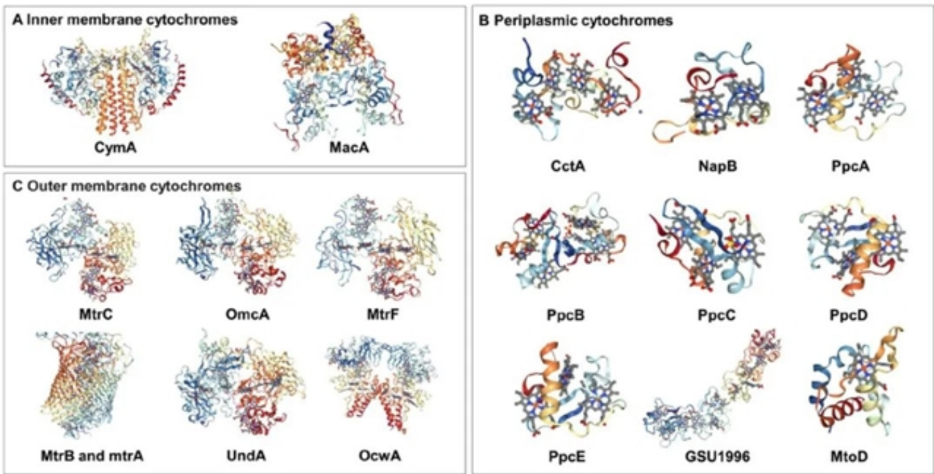
图2. 细胞色素蛋白分类及结构 A.内膜细胞色素; B.周质空间细胞色素；C外膜细胞色素
