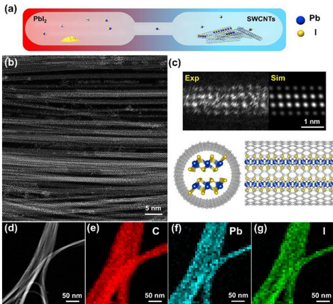
单壁碳纳米管封装碘化铅一维范德华异质结的结构表征
