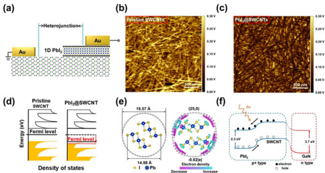
单壁碳纳米管封装碘化铅异质结电子传输机制
