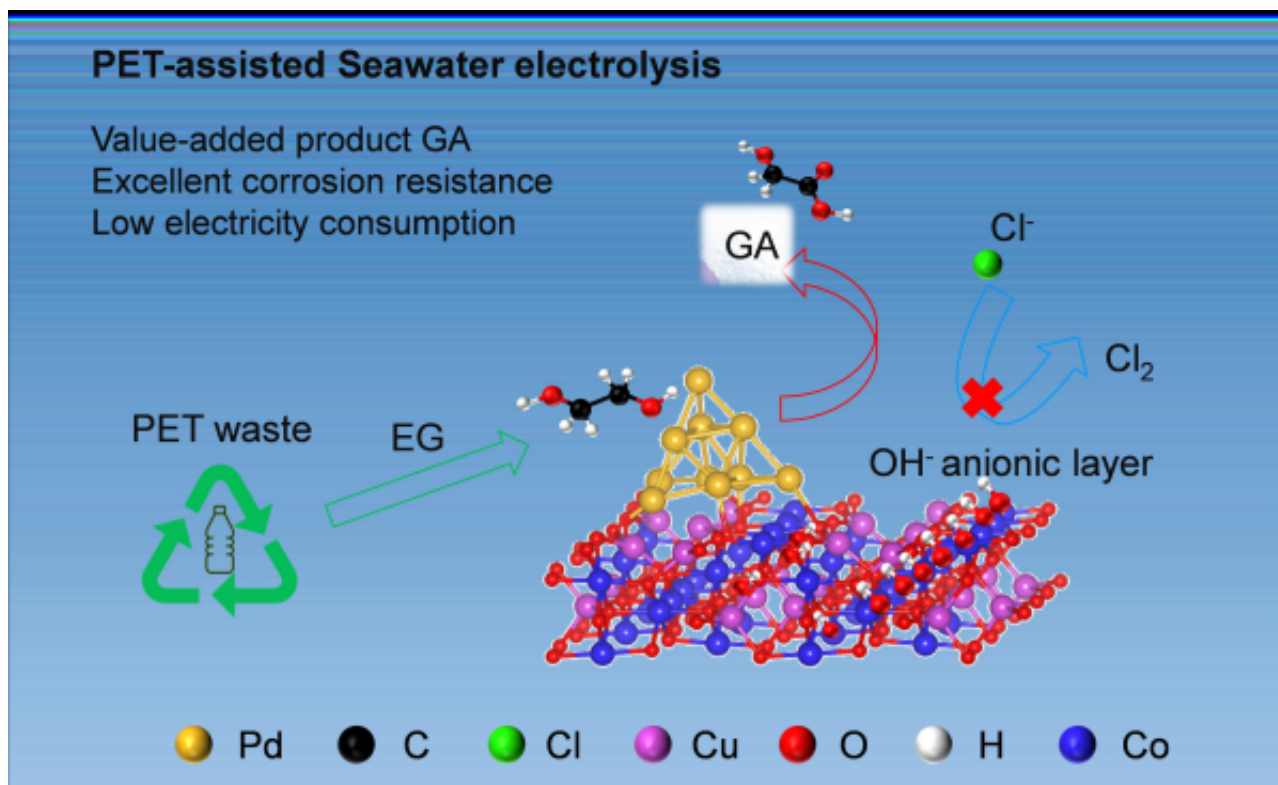
电化学氧化PET耦合海水制氢示意图
