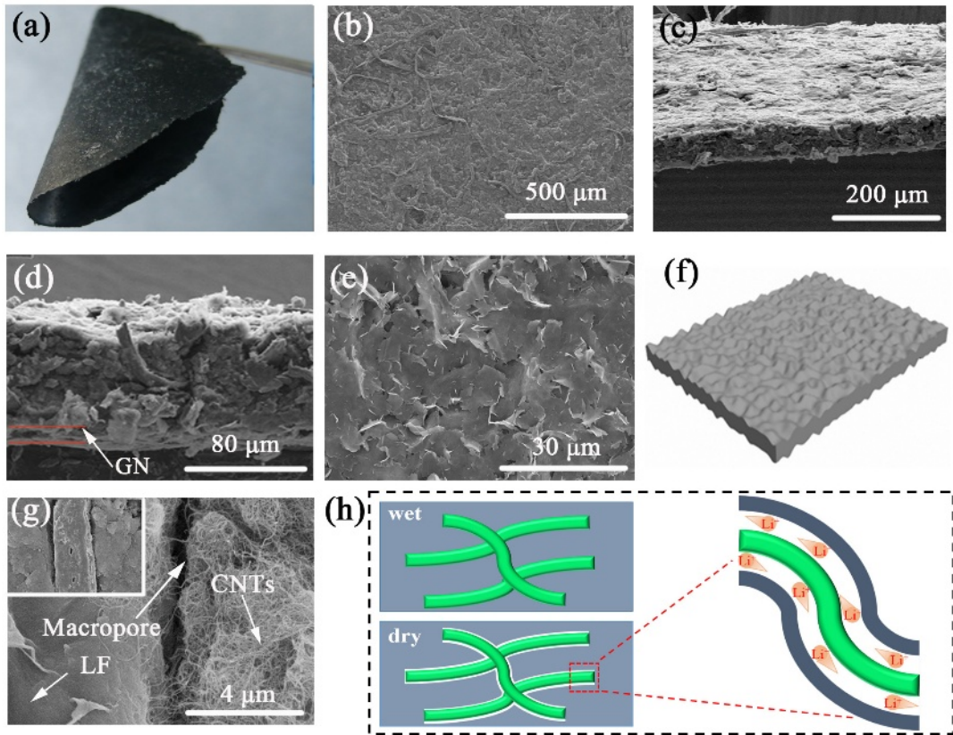
“类钢筋混凝土”柔性载硫体极片及相关结构示意图
