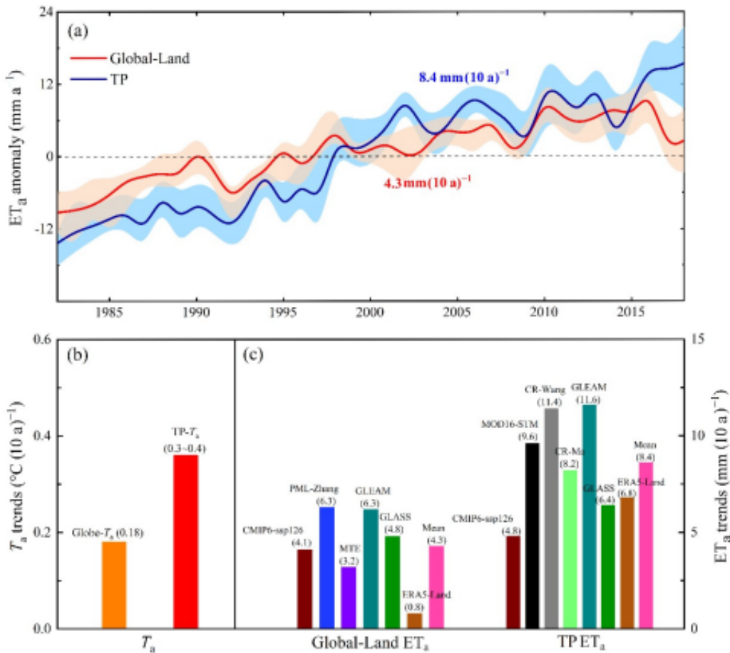
1982-2018年青藏高原蒸散发变化趋势 (a) 和升温速率 (b) 与全球陆地结果的对比，(c) 根据各套蒸散发数据得到的变化速率及集合平均结果
