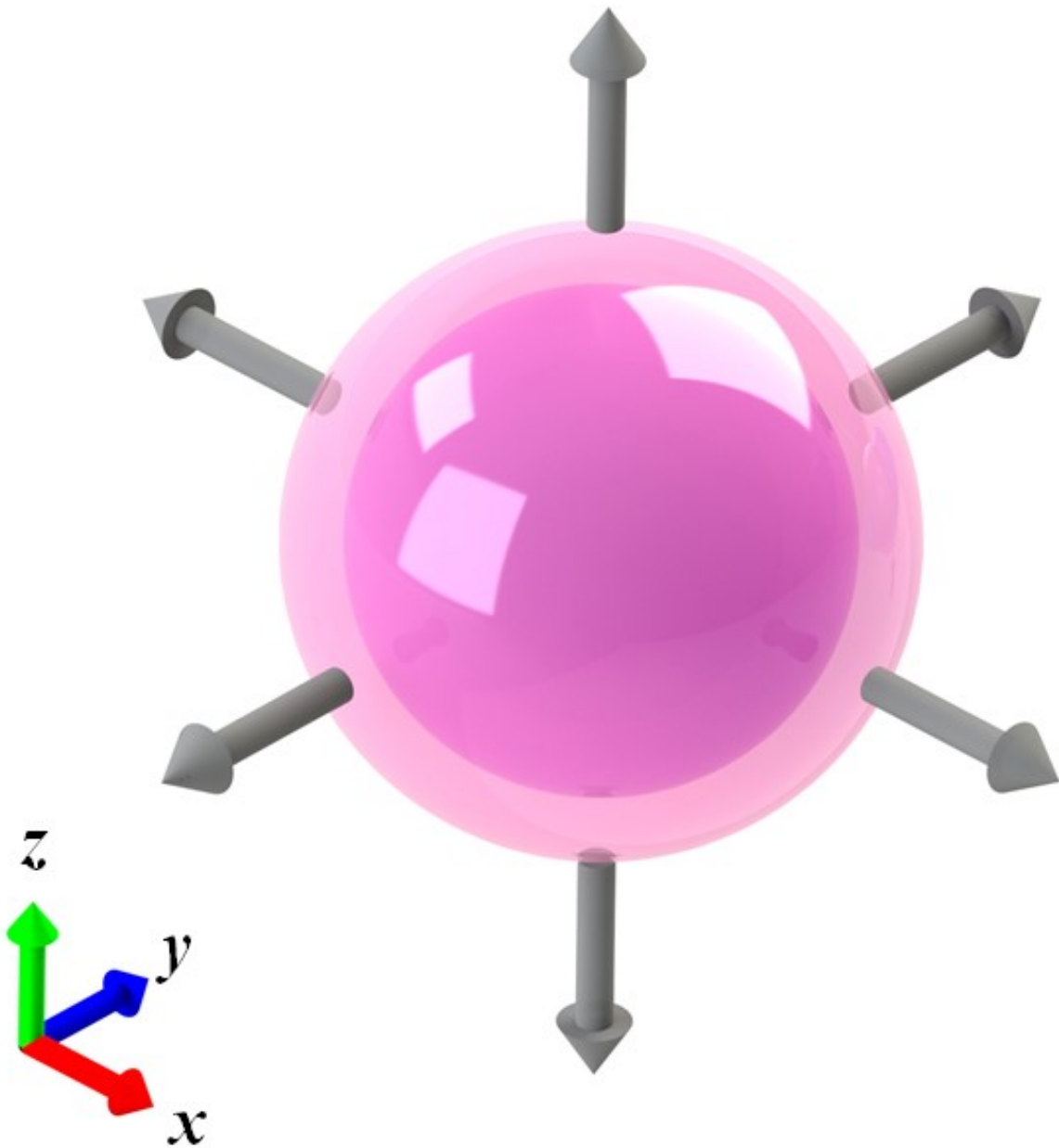
球形么正费米气体示意图
