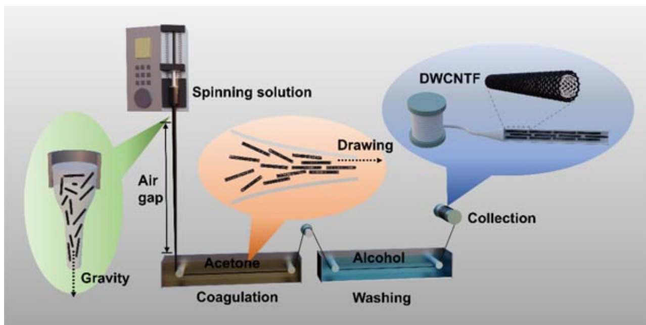
干喷湿纺制备高性能碳纳米管纤维的过程示意图
