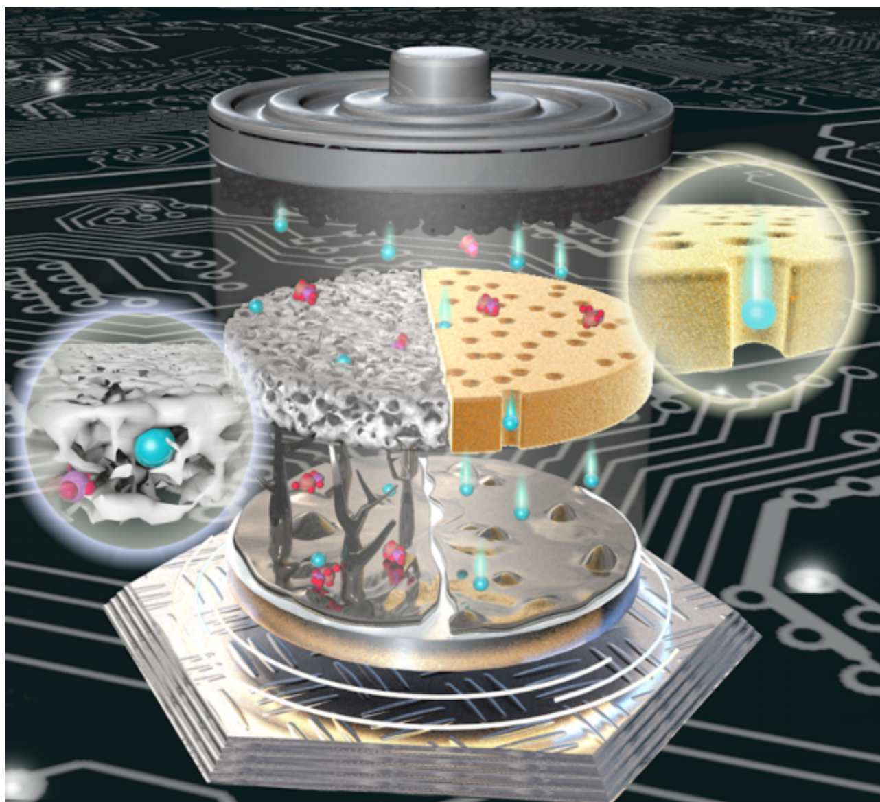
离子管理膜和传统多孔隔膜的离子传输特性和阳极表面锂沉积行为示意图
