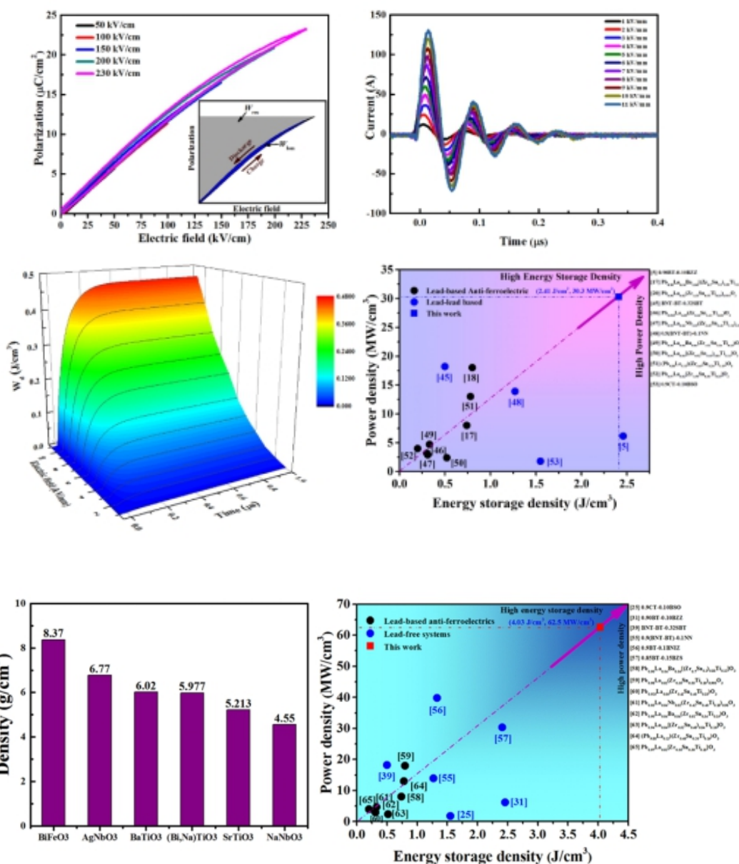
几种典型无铅介质材料体系的体积密度对比图(左)和Na 1-3x BixNbO 3 综合储能特性与文献对比图(右)
