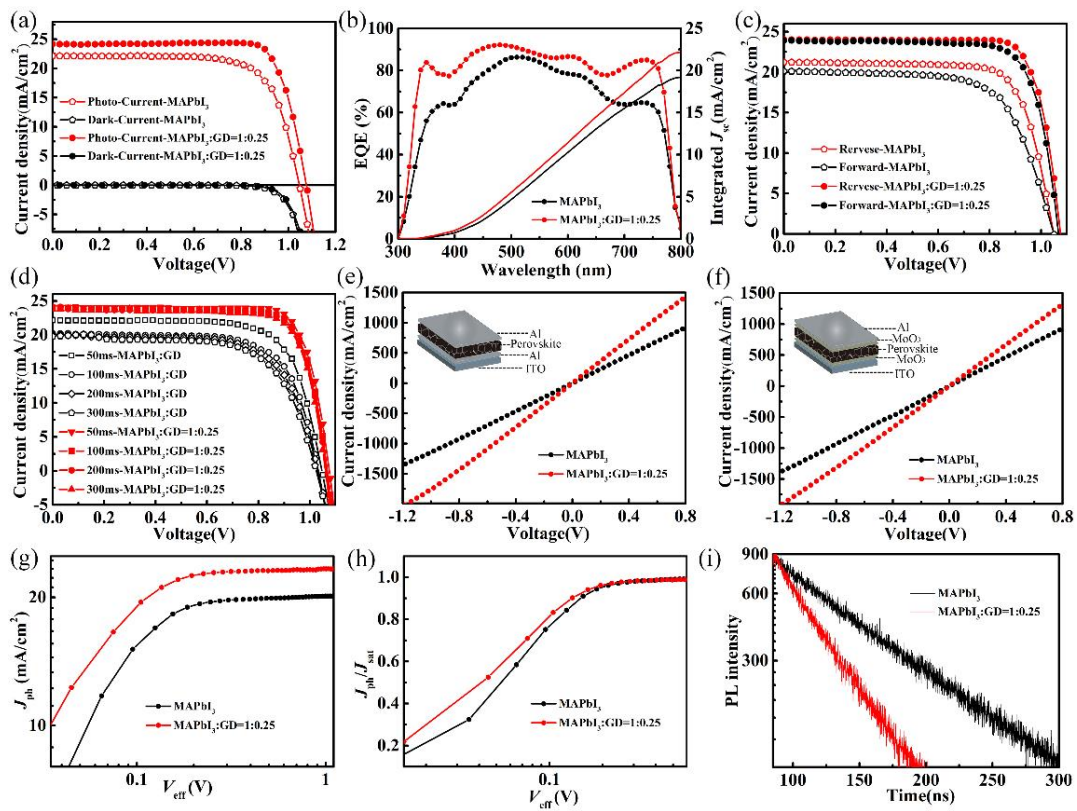
图：石墨炔作为主体材料所制备的钙钛矿器件结构及光电性能
