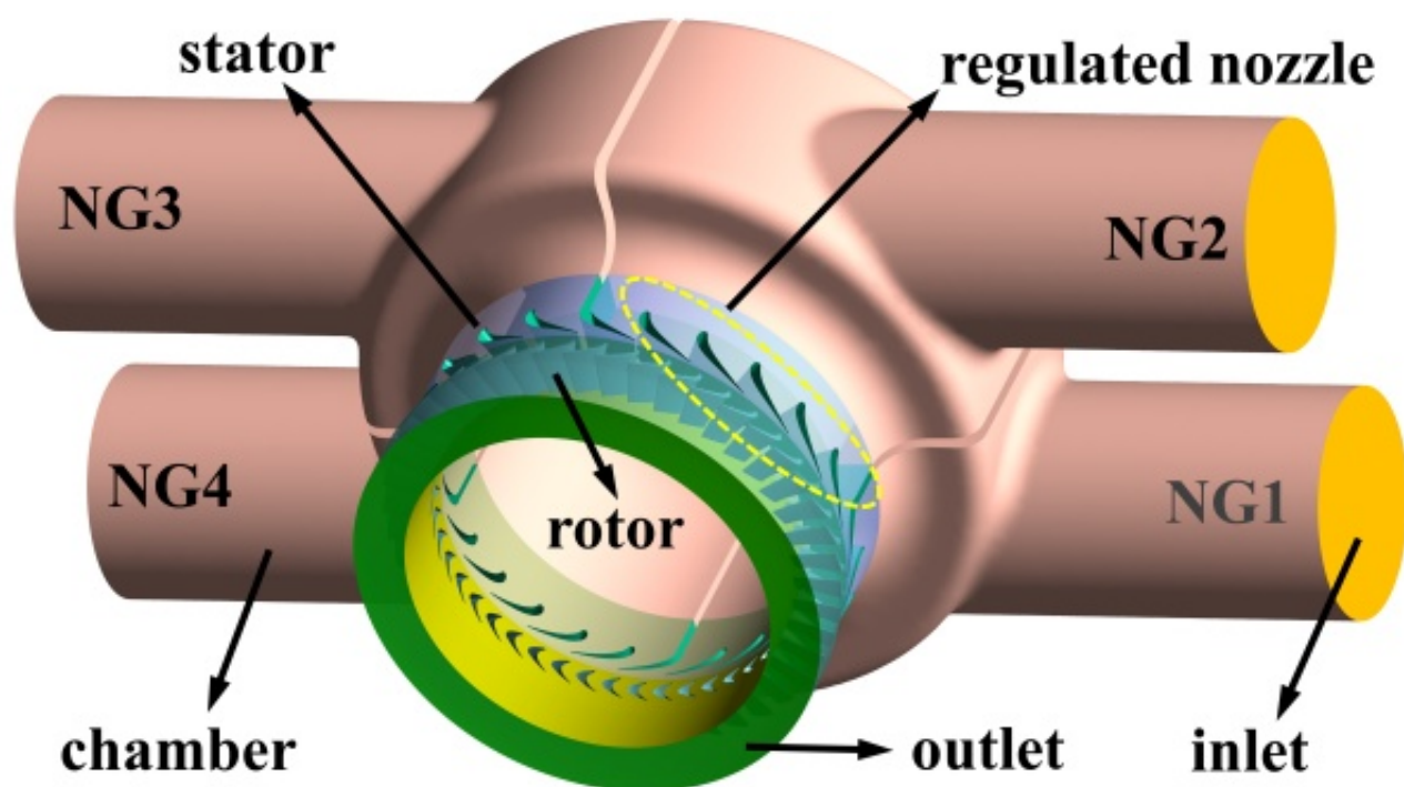
变调节安装角喷嘴配气膨胀机三维模型
