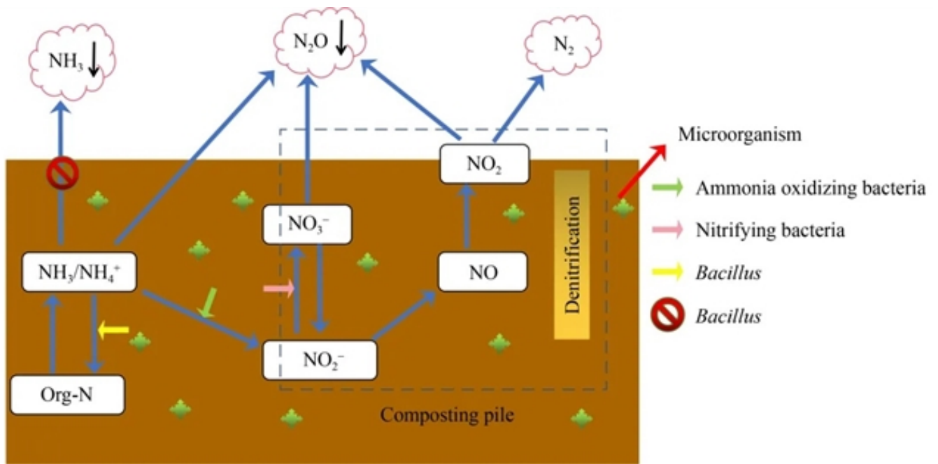
图5 微生物添加剂在堆肥过程减少氮损失的机理。
