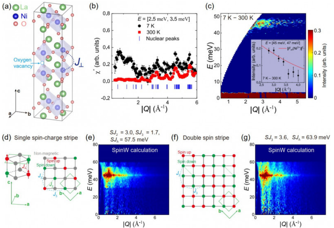
La 3 Ni 2 O 7 的晶体结构与自旋激发谱。(a) La 3 Ni 2 O 7 的晶体结构；(b) 动态磁化率随动量的变化关系；(c) 低温与高温自旋激发的差值；(d) 和 (e) 单自旋-电荷条纹相的自旋排列与相应的自旋激发拟合结果；(f) 和 (g) 双自旋条纹相的自旋排列与相应的自旋激发拟合结果。研究团队供图
