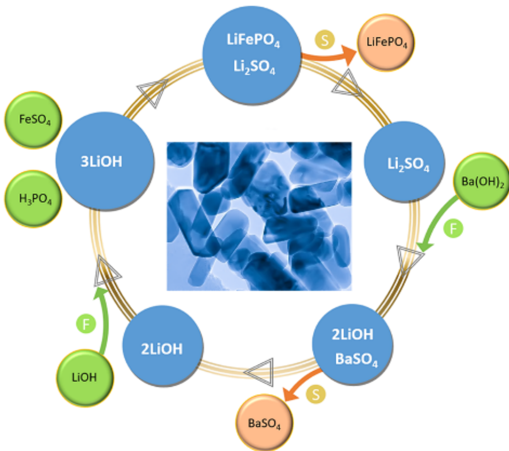
图2 LiFePO 4 纳米晶水热合成路线及锂回收示意图。以LiOH、FeSO 4 和H 3 PO 4 为原料制备纳米LiFePO 4 。用Ba(OH) 2 做沉淀剂与滤液反应，随后进行固液分离，回收LiOH。插图为LiFePO 4 的TEM照片。
