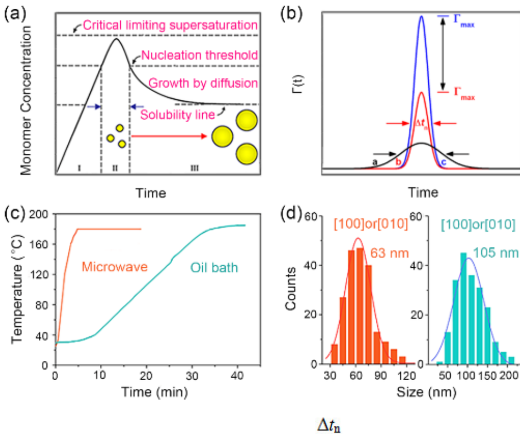
图1 经典的LaMer形核和生长机制以及实验结果。(a)经典LaMer机理，颗粒在溶液中成核和生长过程中单体浓度变化的示意图。(b)三个具有高斯分布的形核函数。形核函数的宽度( \Delta t_n )对应形核时间窗口。(c)微波加热和油浴加热两种加热模式下的原位温度与时间曲线。(d)由两种不同的加热模式制备的 \text{LiFePO}_4 沿[100]或[010]方向的尺寸统计。微波加热的尺寸为63nm，而在常规油浴加热的情况下，尺寸为105nm。
