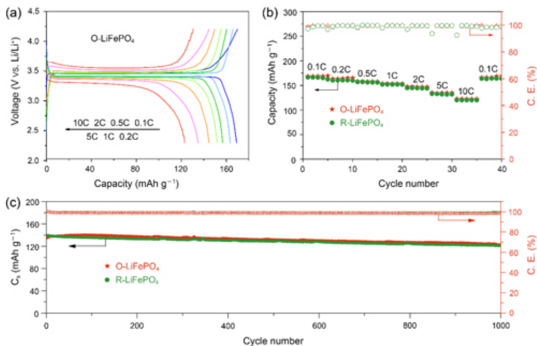
图4 原始的O-LiFePO 4 /C和回收的R-LiFePO 4 /C的电化学性能曲线。(a)O-LiFePO 4 /C在0.1 – 10C不同倍率范围内的典型充放电曲线。(b)倍率性能。(c)O-LiFePO 4 /C和R-LiFePO 4 /C在3C倍率下的长循环稳定性。3C对应的充电或放电时间为20分钟。
