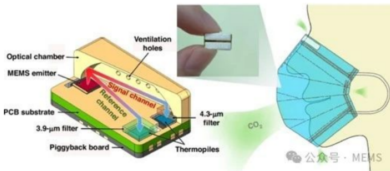
超小型双通道集成CO 2 红外气体传感器原理图及可穿戴呼吸检测装置
