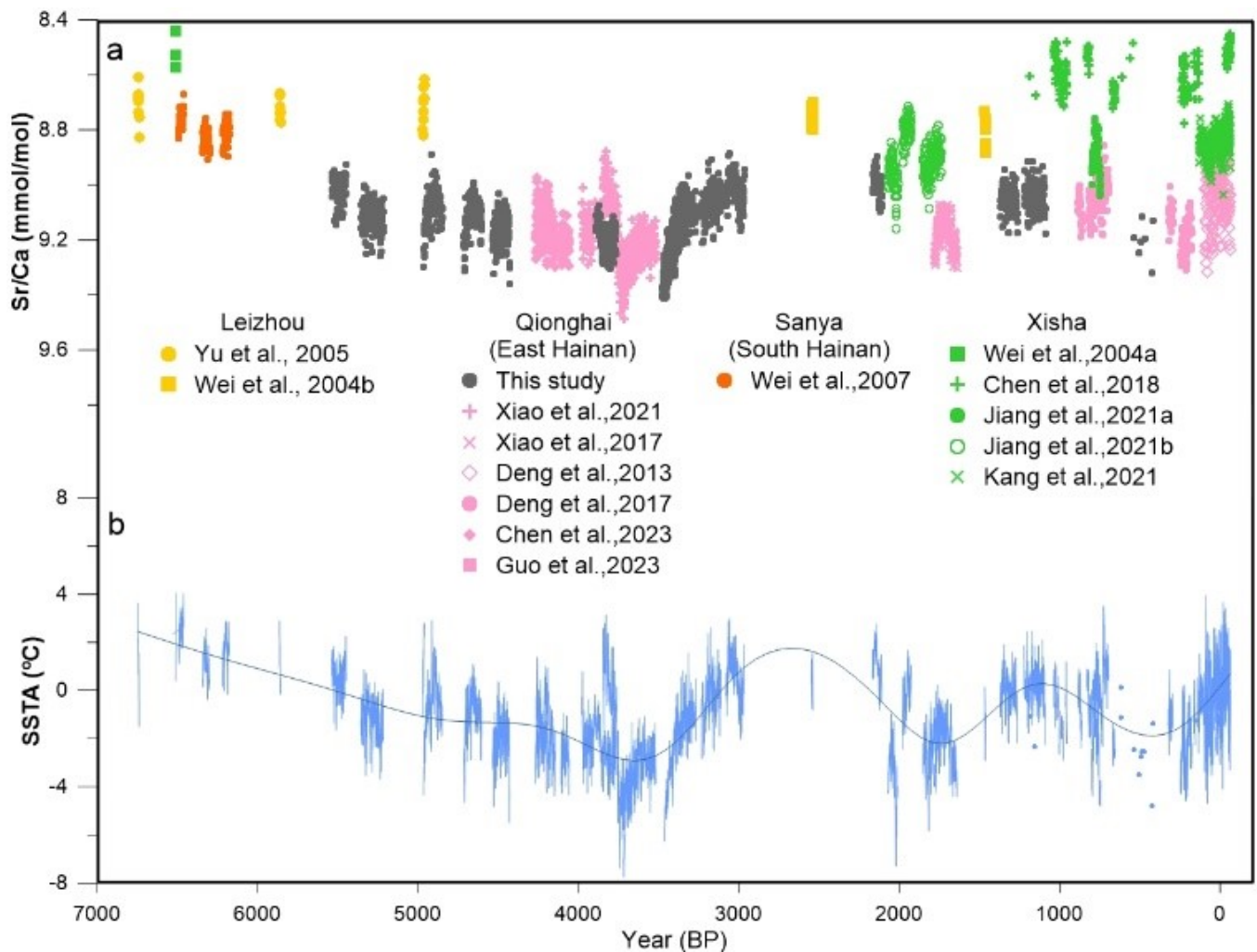
南海北部珊瑚Sr/Ca-SSTA记录。研究团队供图
